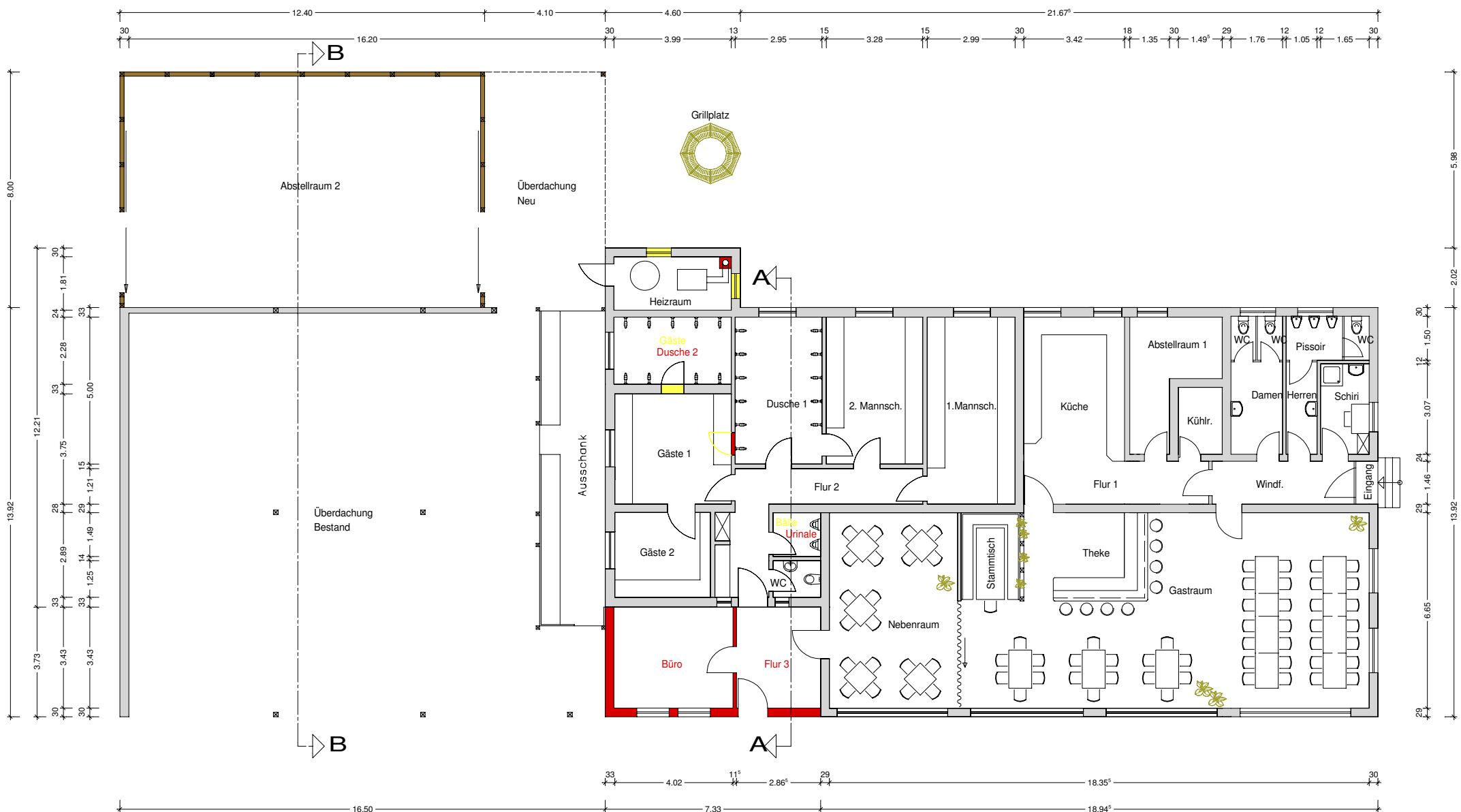
Erdgeschoss M 1:175
