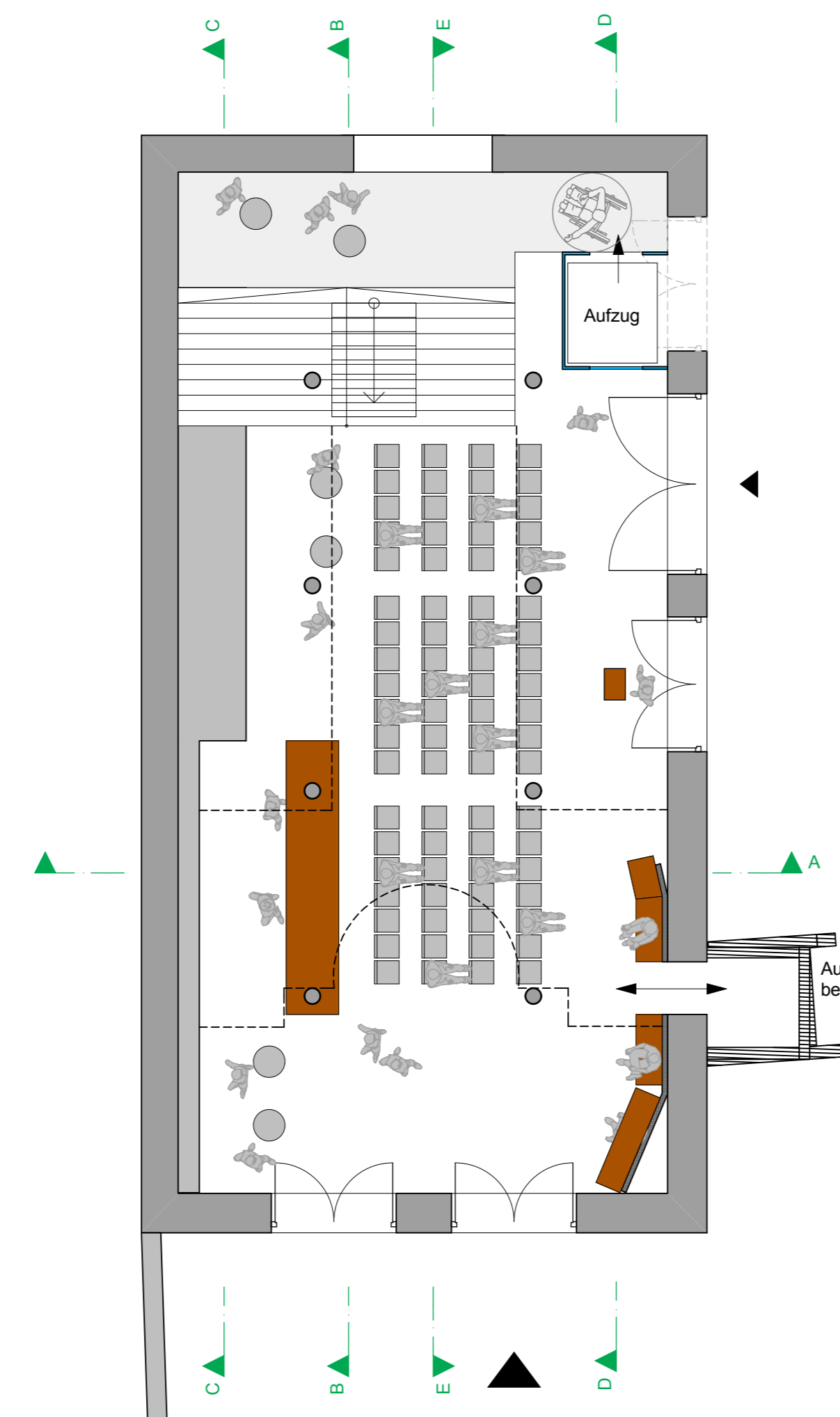
EINGANG / ERDGESCHOSS
