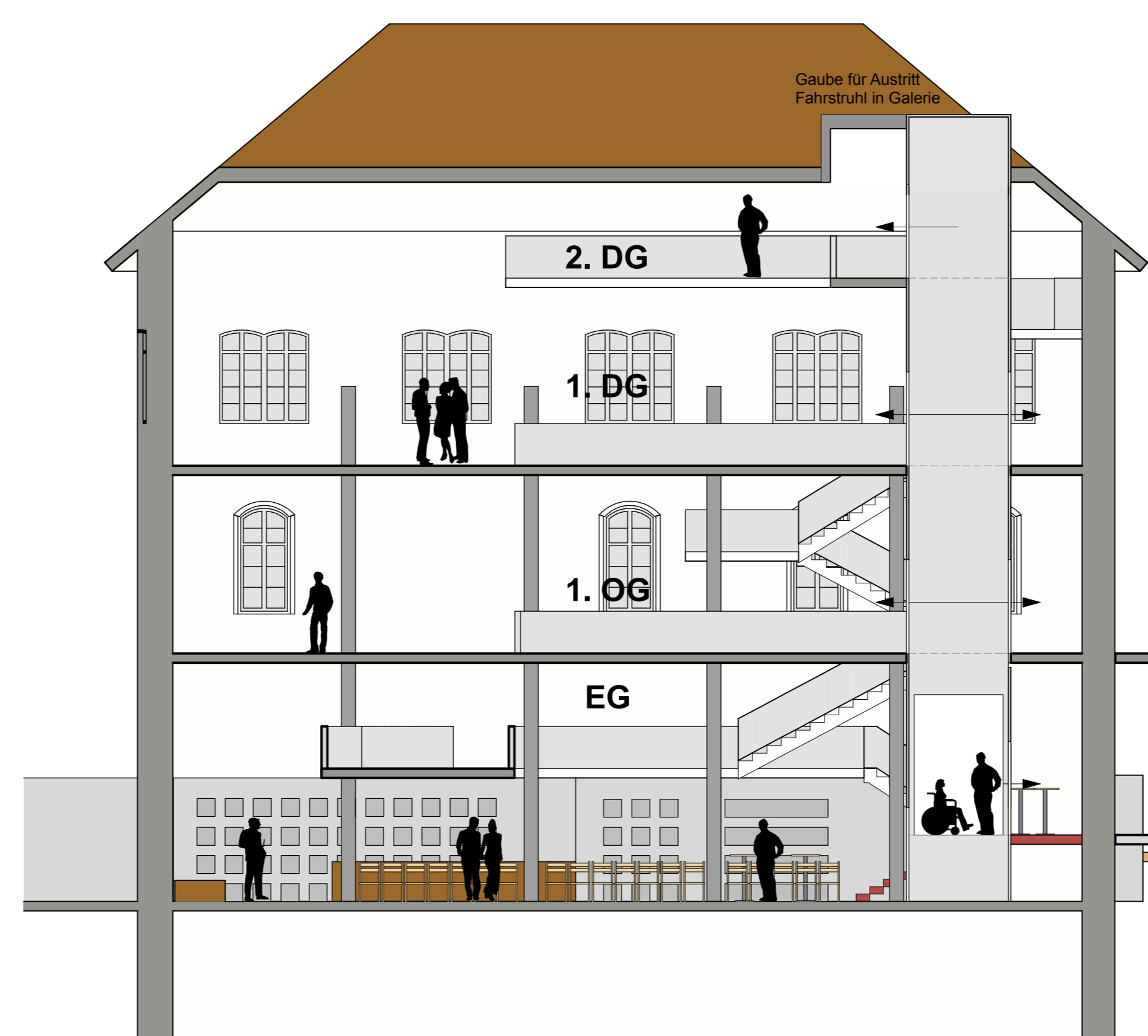
SCHNITT D
