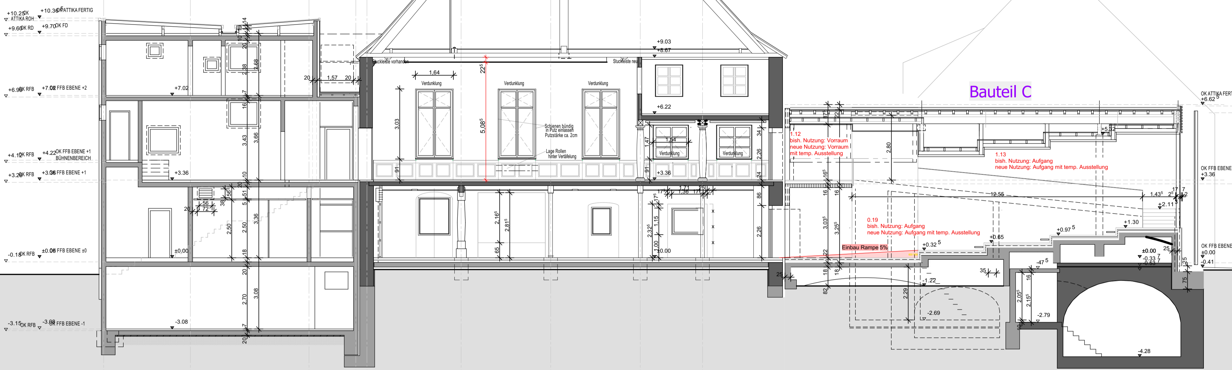
SCHNITT A-A
