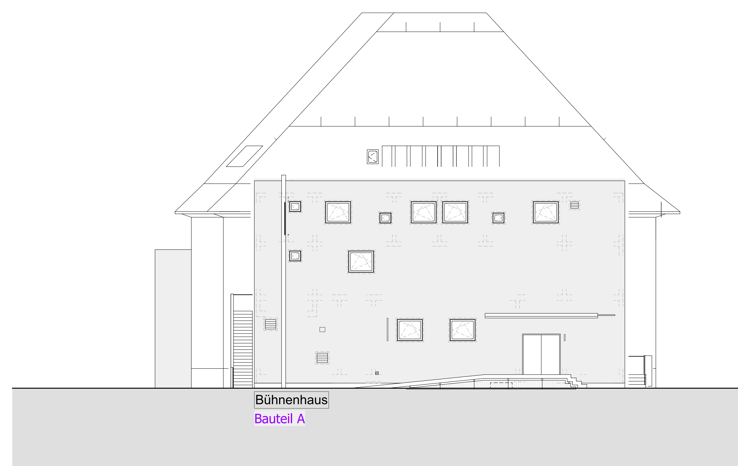
ANSICHT SÜD-WEST
