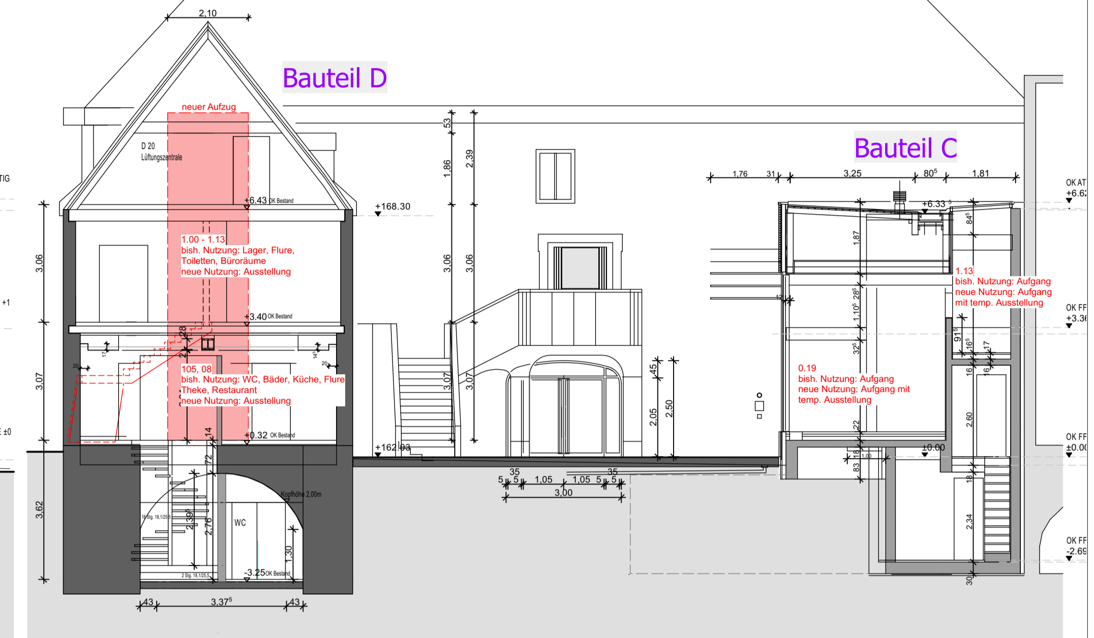
SCHNITT B-B
