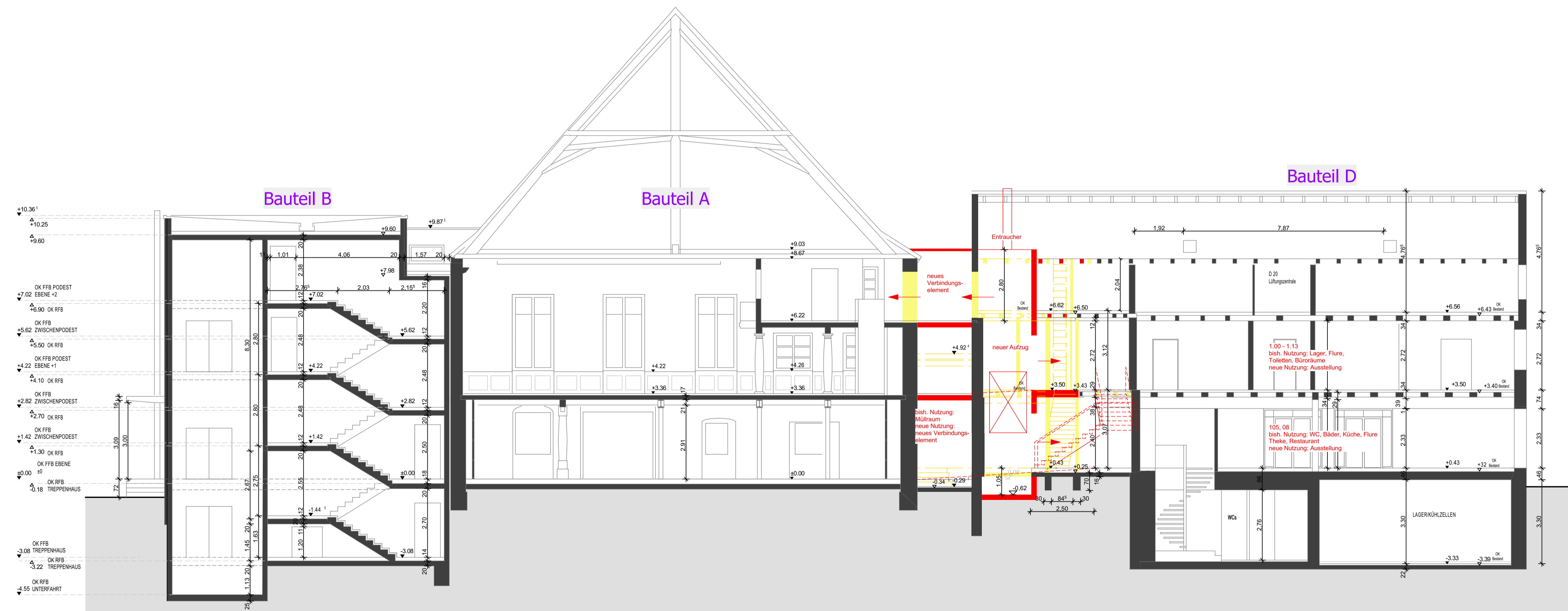
SCHNITT D-D
