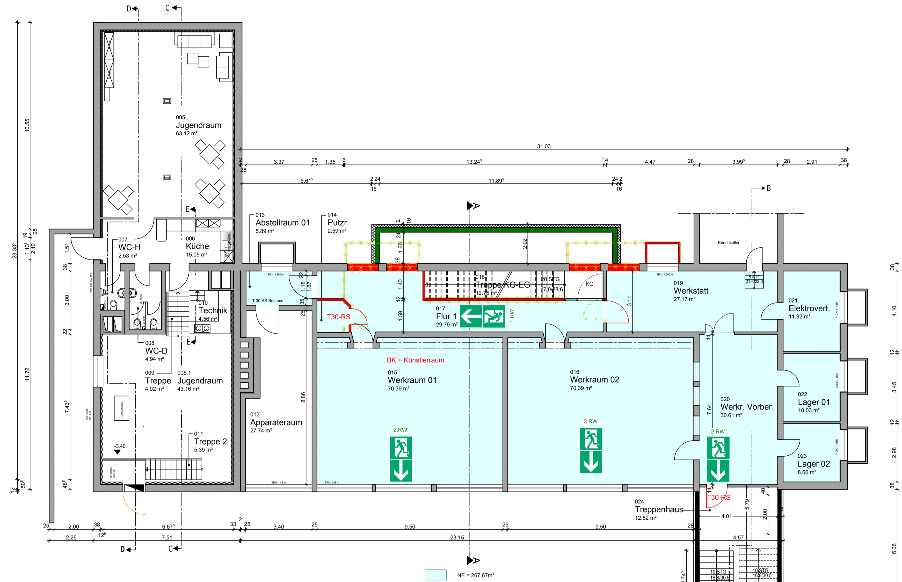
Kellergeschoss Verwaltung Geb. 119 --- 1.Ebene---Brandschutz BA 2019
