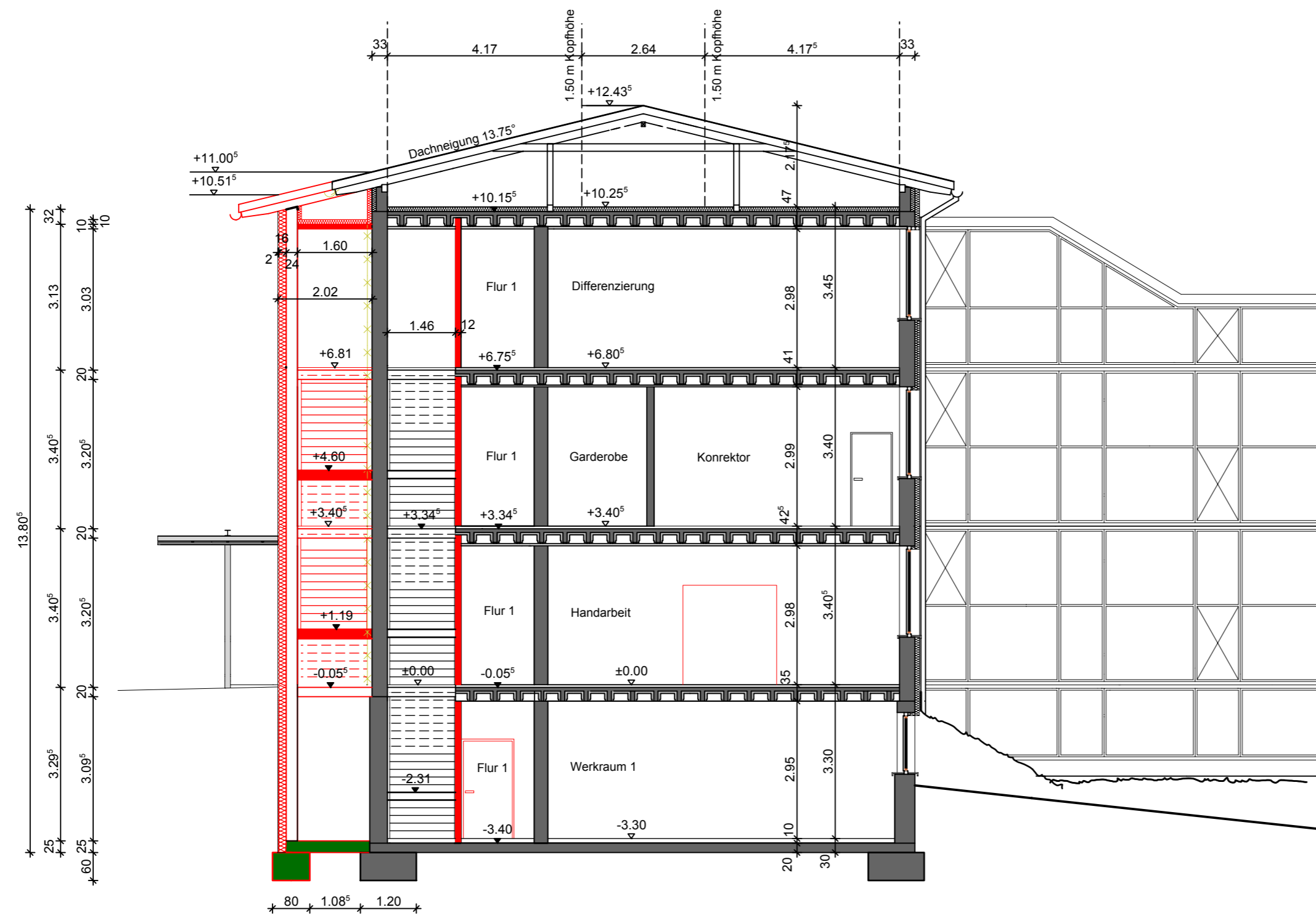
Schnitt A-A - Geb.119 VW
