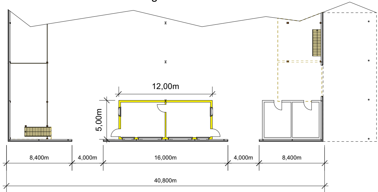
Draufsicht Lagerhalle
