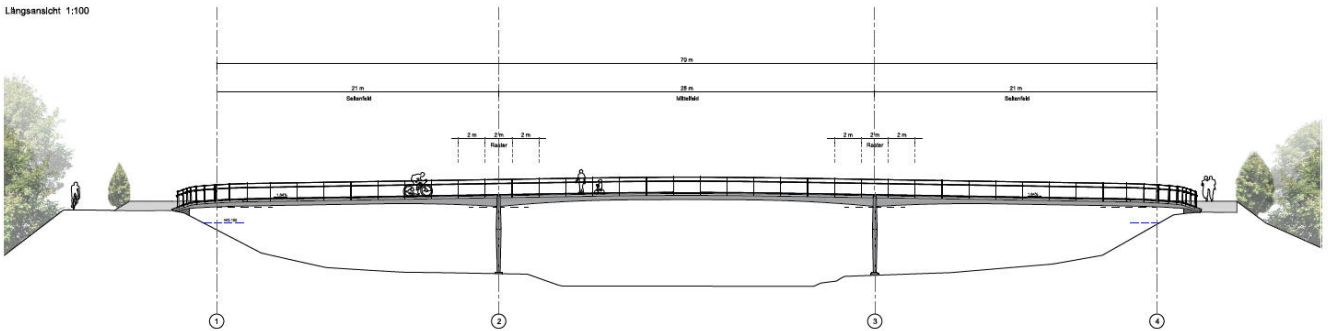
Längsansicht 1:100
