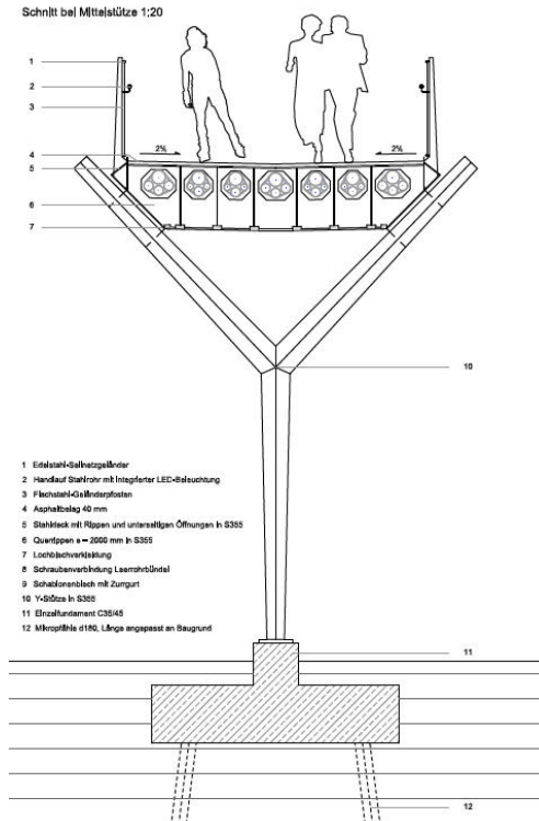
Schnitt bei Mittelstütze 1:20
