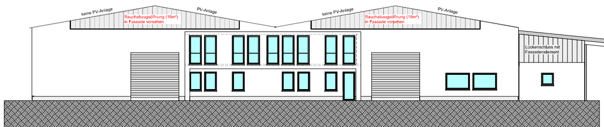
Nordansicht
