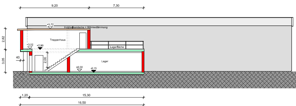
Schnitt A-A
