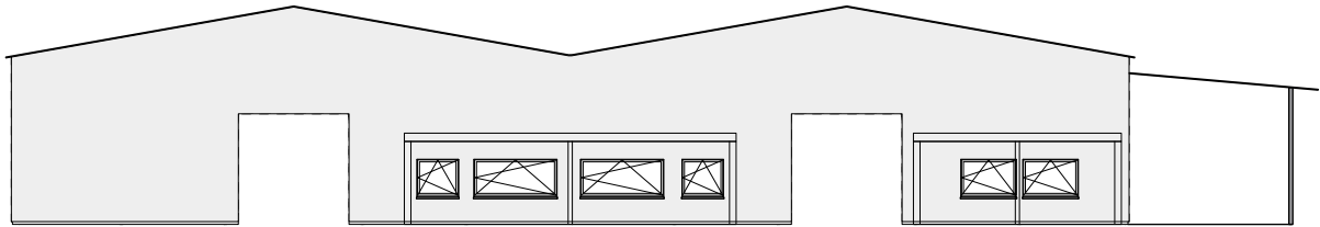
Vorderansicht Lagerhalle
