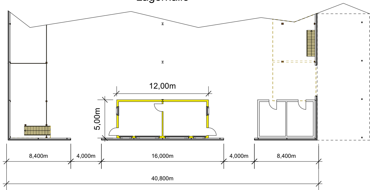
Draufsicht Lagerhalle
