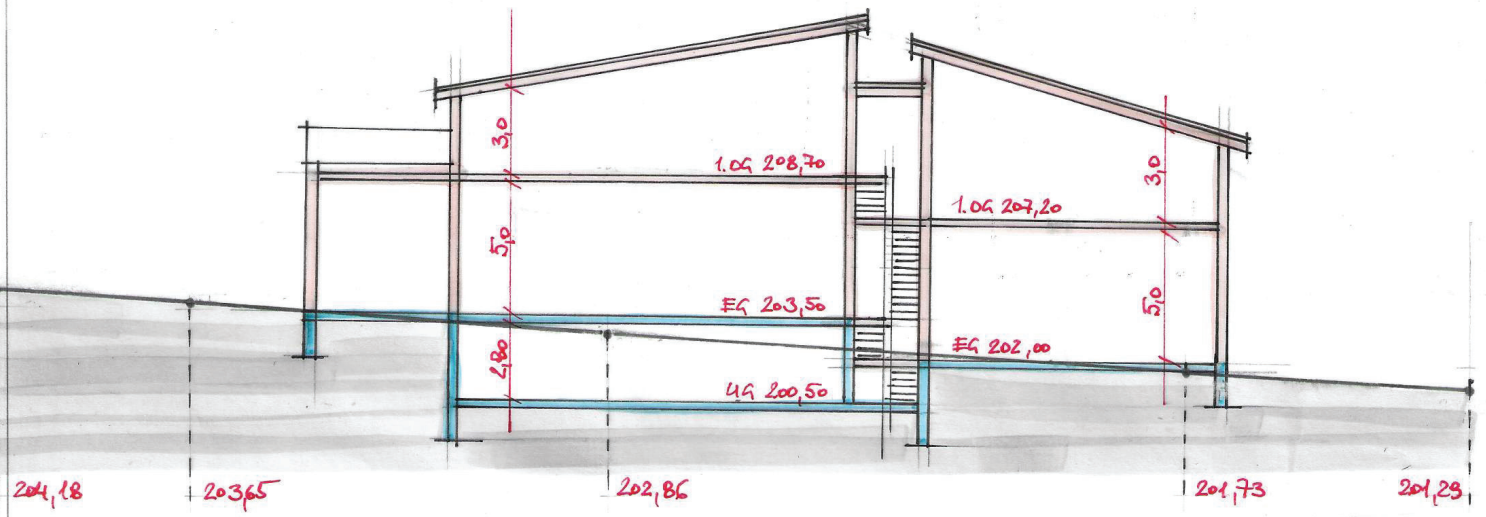
QUERSCHNITT
