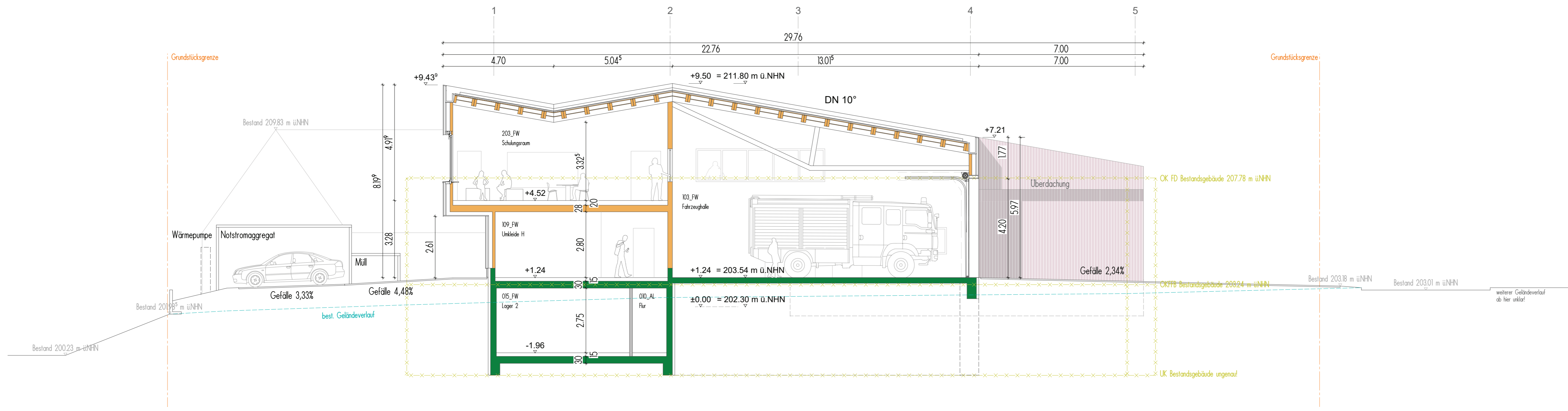
Schnitt A-A_Schulungsraum | Fahrzeughalle Feuerwehr
