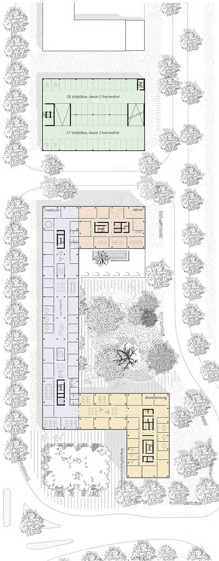
grundriss 1. obergeschoss/regelgeschoss
