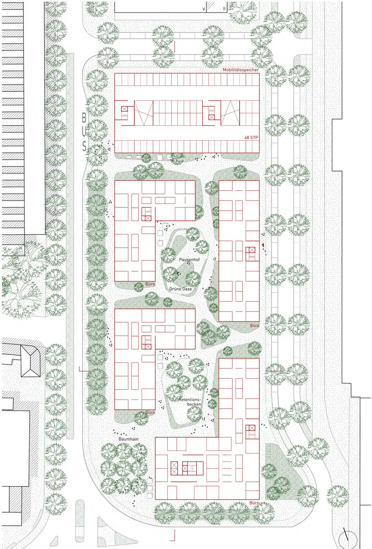
Grundriss OG
