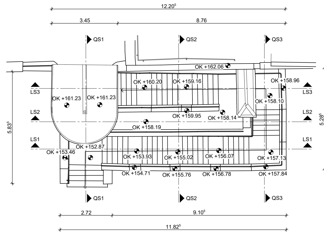
Draufsicht
